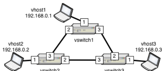
図 1 演習対象のネットワーク
