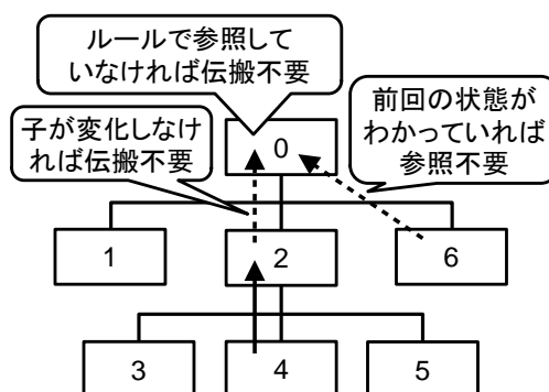
図8 ロールアップの通信削減方式
