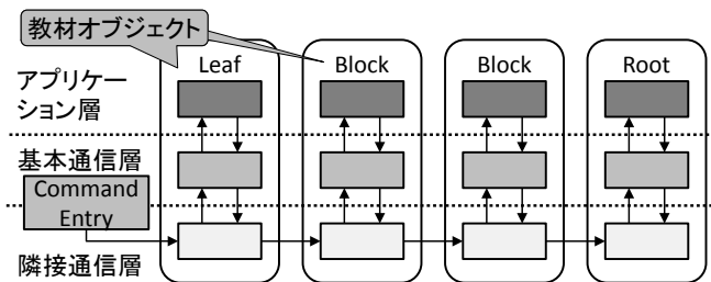
図 3 レイヤーデザインパターンによる教材オブジェクト間通信
